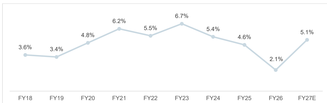
CPI trendline
